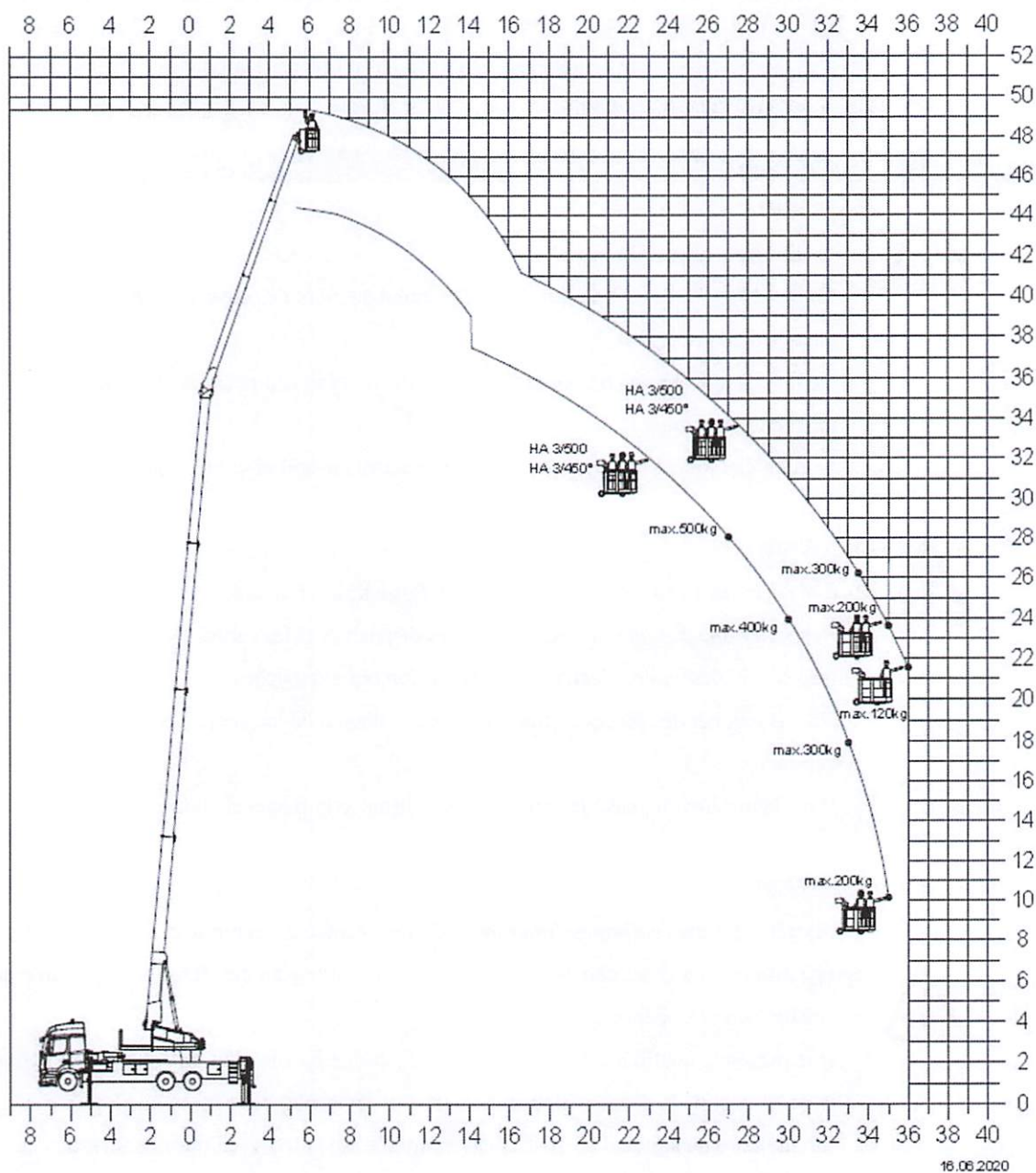
Fig. 4-5 Plage de travail en mode plateforme élévatrice K 1003 RSX / RHX Les valeurs varient en fonction du véhicule porteur.
