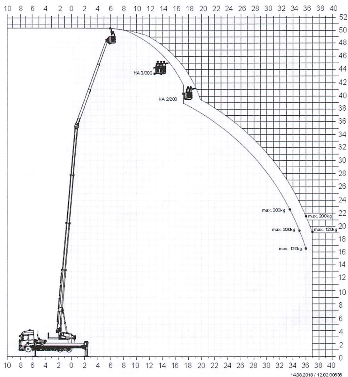
Fig. 4-4 Plage de travail en mode plateforme élévatrice K 1003 RSX / RHX Les valeurs varient en fonction du véhicule porteur.
